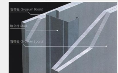
Exterior Wall Type 8 外墙类型8
