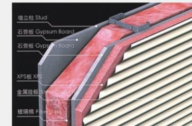
Exterior Wall Type 5 外墙类型5
