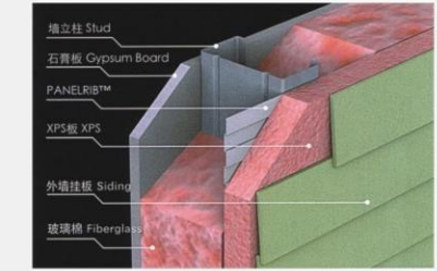
Exterior Wall Type 4 外墙类型4
