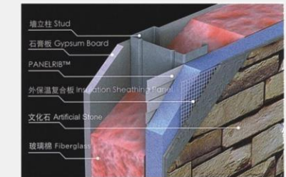
Exterior Wall Type 6 外墙类型6
