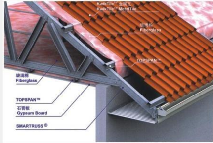
Roofing Type 1 屋面类型1
